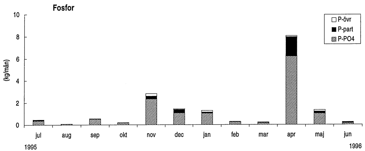
Figur 3. Månadsvärden av vattenföring (1000*m³/mån) och kväve- och fosfortransporter (kg/mån) i Barlingbo avrinningsområde 1995/96.
