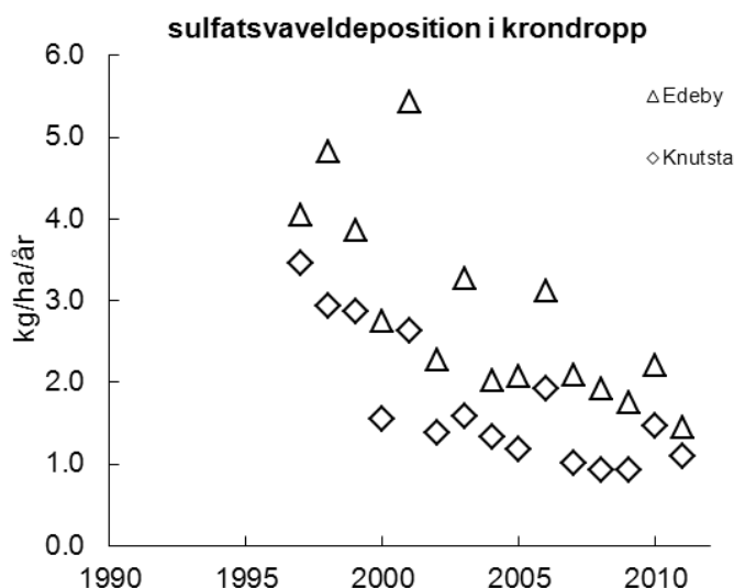
Figur 2. Nedfall av sulfatsvavel i krondropp exklusive bidrag från havssalt vid olika platser i Södermanlands län, uppmätt inom Krondroppsnetet.
