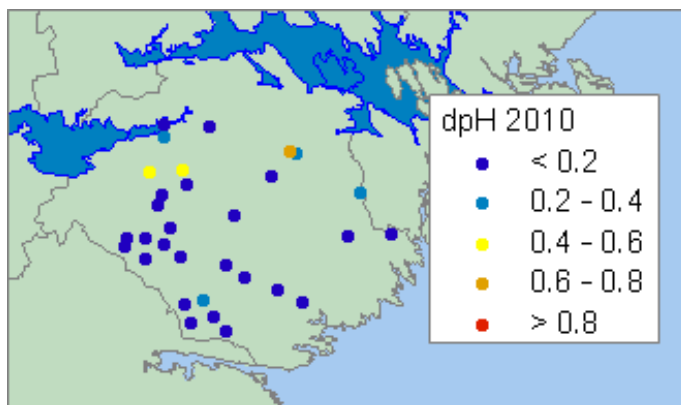
Figur 5. pH-förändring sedan förindustriell tid (dpH) i sjöar 2010, baserat på MAGIC-biblioteket. En sjö räknas som antropogent försurad om pH som årsmedian har sjunkit med minst 0,4 enheter sedan förindustriell tid (dpH > 0,4), vilket markeras med gula, orange och röda symbolerna på kartan. Analysen inkluderar kalkade försurade sjöar baserat på beräknad vattenkemi om man inte hade kalkat.
