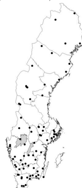
Figur 1. Krondroppsnätet under 2010/11. Samordnade mätningar av luftföroreningar i skogliga observationsytor.
