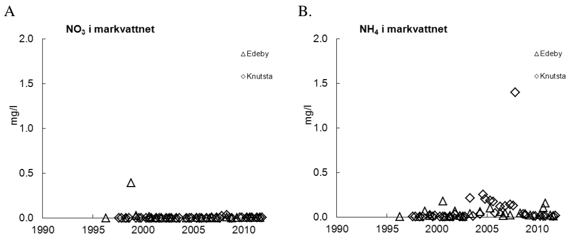
Figur 10. Halterna av nitrat (A) och ammonium (B) i markvattnet på 50 cm djup vid olika platser i Södermanlands län, uppmätt inom Krondroppsnätet.
