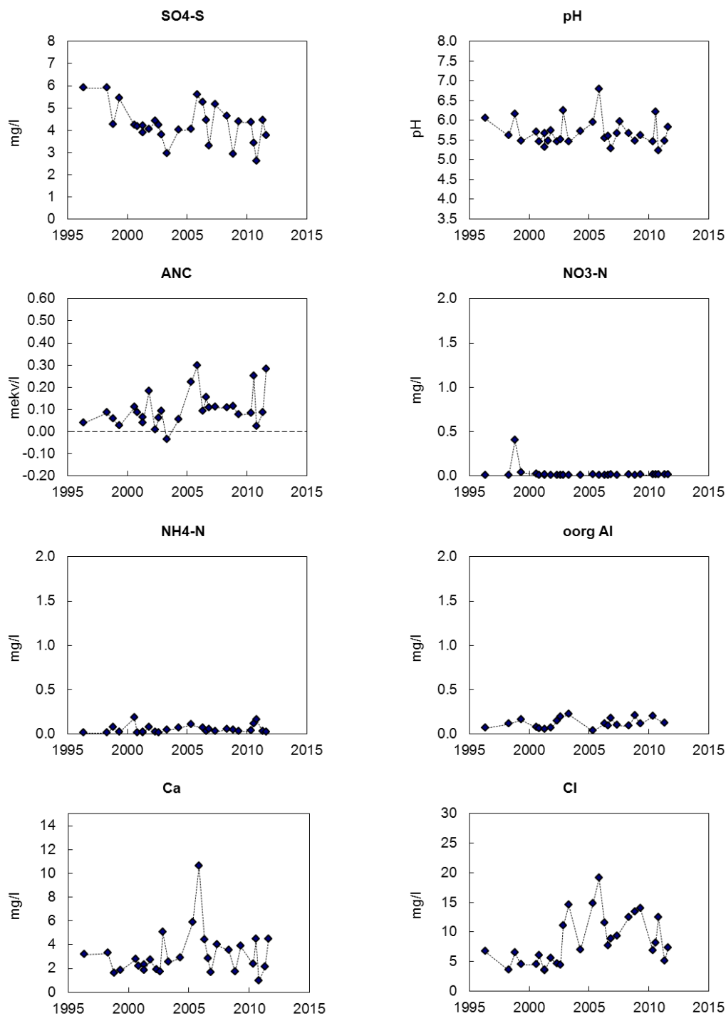
Figur B1:2. Markvattenkemi vid Edeby, D 11. Sulfatsvavel ( \text{SO}_4\text{-S} ); pH; markvattnets syraneutraliserande förmåga (ANC); nitratkväve ( \text{NO}_3\text{-N} ); ammoniumkväve ( \text{NH}_4\text{-N} ); oorganiskt aluminium (oorg Al); kalciumhalt ( \text{Ca}^{2+} ); kloridhalt (Cl). Saknade värden innebär oftast att marken varit för torr. Trendanalys har genomförts med hjälp av Seasonal-Kendall metodik och signifikansnivåer anges, ovanför respektive diagram, i de fall där signifikanta trender påvisats.
