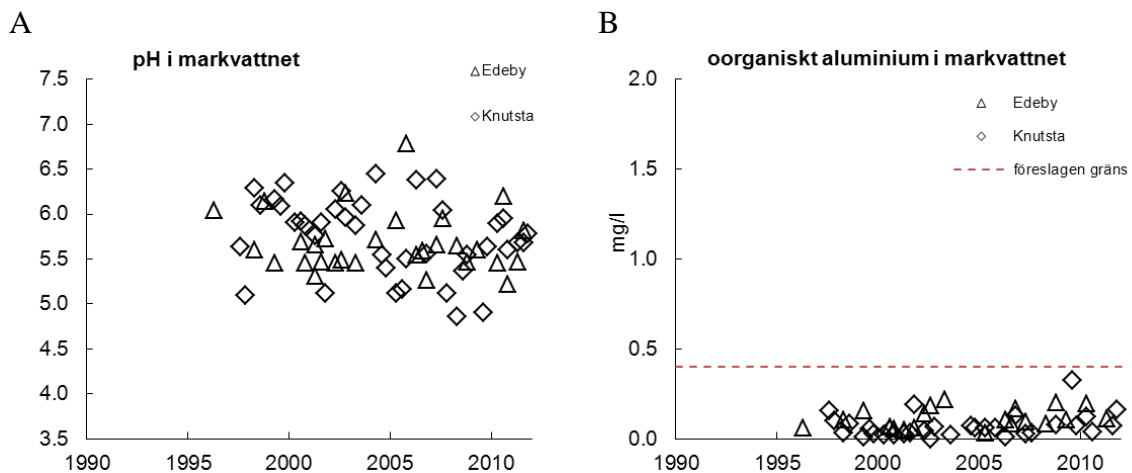
Figur 4. pH (A) och halten oorganiskt aluminium (oorg-Al) (B) i markvattnet på 50 cm djup vid olika platser i Södermanlands län, uppmätt inom Krondroppsnetet.
