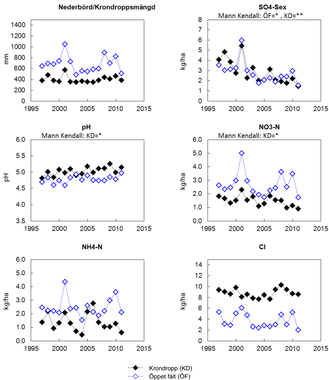
Figur B1:1. Årliga värden (hydrologiskt år) för depositionen via krondropp och över öppet fält vid Edeby, D 11. I figuren visas uppmätt nederbörd över öppet fält samt krondroppsmängder, uttryckt som mm. Deposition redovisas sedan mätningarna påbörjades för ett urval av ämnen: sulfatsvavel utan havssaltsbidrag (SO 4 -S ex), pH; nitratkväve (NO 3 -N); ammoniumkväve (NH 4 -N); kloridjoner (Cl). ÖF, öppet fält; KD, krondropp. Trendanalys har genomförts med hjälp av Mann- Kendall metodik och signifikansnivåer anges, ovanför respektive diagram, i de fall där signifikanta trender påvisats.
