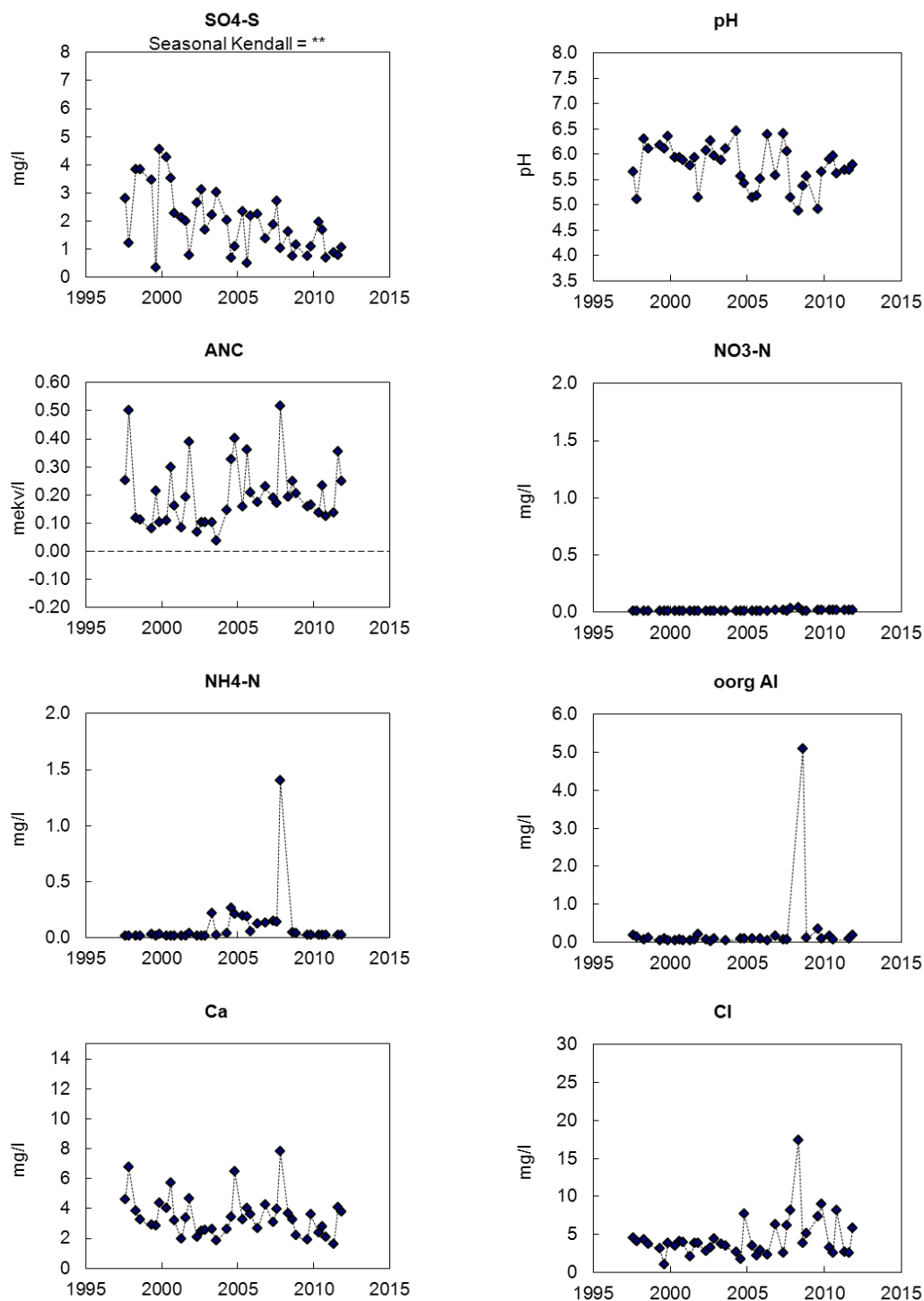
Figur B1:4. Markvattenkemi vid Knutsta, D 14 . Sulfatsvavel (SO 4 -S); pH; markvattnets syraneutraliserande förmåga (ANC); nitratkväve (NO 3 -N) samt ammoniumkväve (NH 4 -N), oorganiskt aluminium (oorg Al); kalciumhalt (Ca 2+ ), samt klorid (Cl). Saknade värden innebär oftast att marken varit för torr. Trendanalys har genomförts med hjälp av Seasonal- Kendall metodik och signifikansnivåer anges, ovanför respektive diagram, i de fall där signifikanta trender påvisats.
