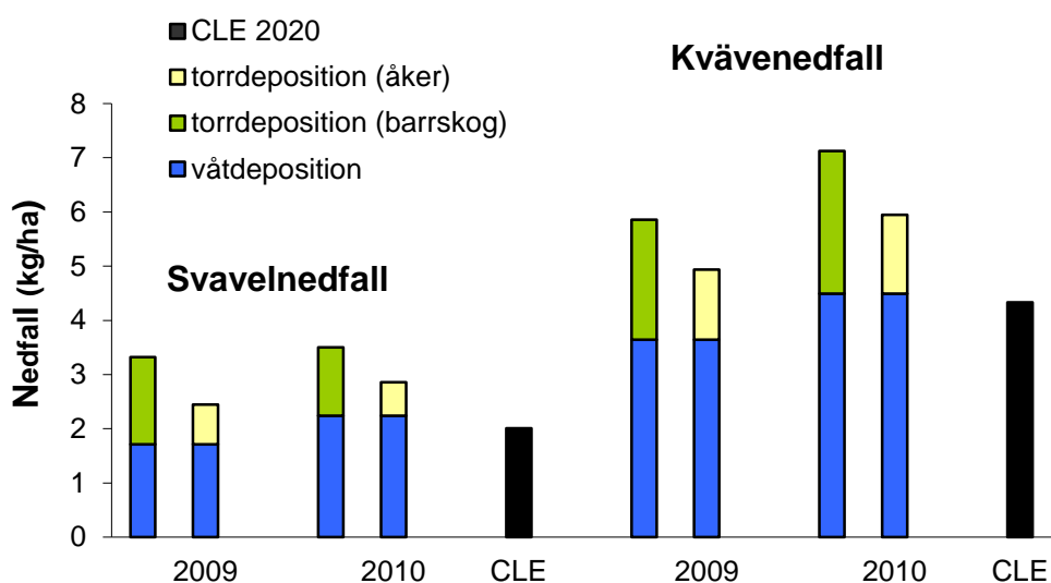
Figur 11. Modellberäknat nedfall av antropogent svavel och oorganiskt kväve (kg per hektar och kalenderår) i Södermanlands län, fördelat på våt- respektive torrdeposition under 2009-2010 och år 2020 enligt CLE-scenariet, modellerat med MATCH-Sverige-modellen. De nedre staplarna anger våtdepositionen och de övre staplarna anger torrdepositionen (till barrskog eller åkermark).
