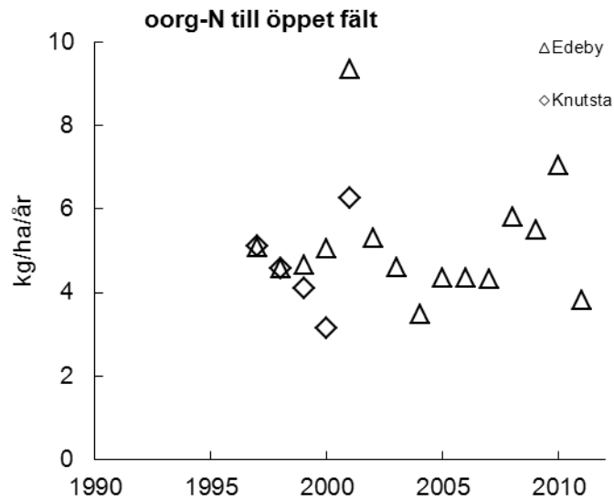
Figur 8. Nedfall av oorganiskt kväve ( \text{NO}_3 + \text{NH}_4 ) med nederbörden till öppet fält vid Edeby och Knutsta i Södermanlands län, uppmätt inom Krondroppsnetet.
