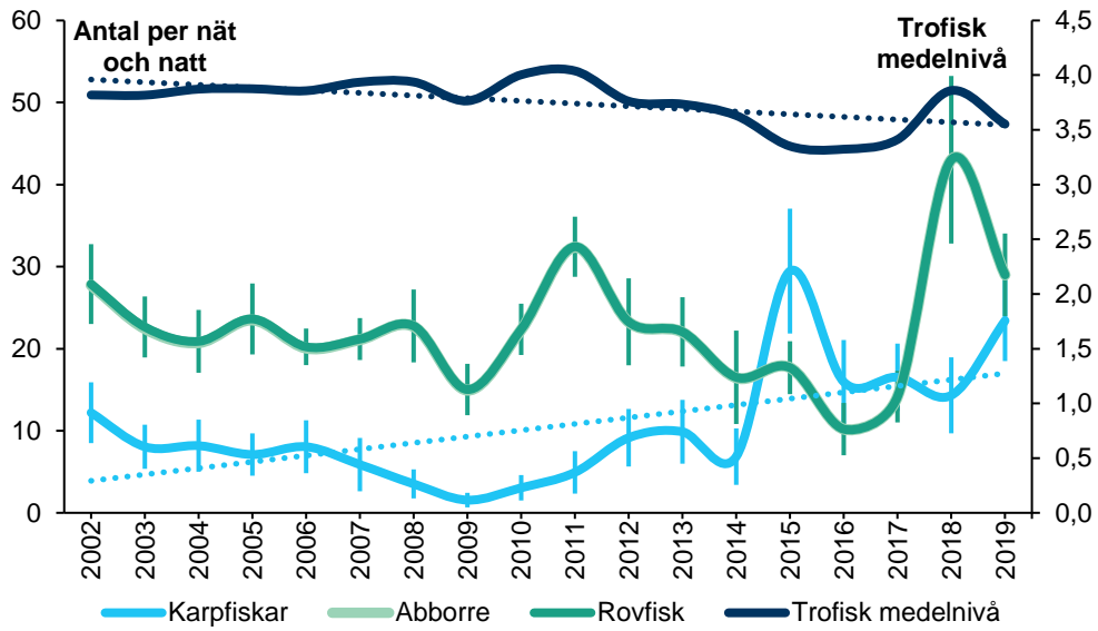
Figur 6. Fångst per nät och natt av rovfiskar, abborre och karpfiskar, samt trofisk medelnivå i provfiskefångsten. Graferna för abborre och rovfisk sammanfaller eftersom abborren är den överlägset mest dominerande rovfisken i provfiskefångsten. Vertikala linjer anger 95 % konfidensintervall. Streckade linjer anger statistiskt säkerställda trender över tid.
