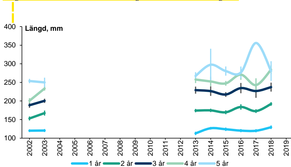
Figur 7. Medellängd av abborrhonor åldrar 1–4 år från Lagnö. Vertikala linjer anger 95 % konfidensintervall. Ingen åldersanalys genomfördes 2004–2012 och 2019.
