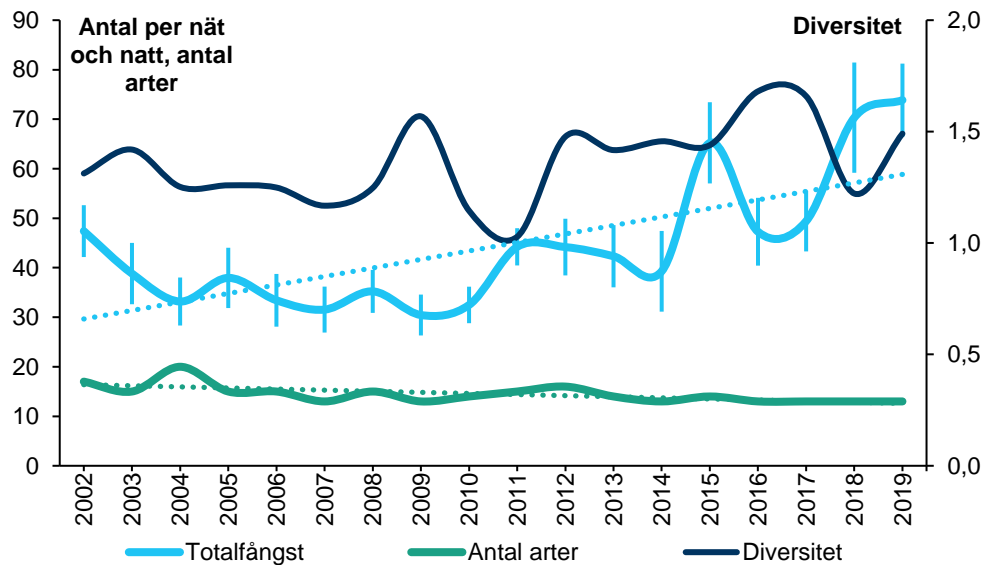
Figur 4. Totalfångst (antal per nät och natt), totala antalet fångade arter, samt diversitet hos provfiskefångsten. Vertikala linjer anger 95 % konfidensintervall. Streckade linjen anger statistiskt säkerställd trend över tid. Diversitet är beräknad som Shannon-Wiener diversitetsindex över hela årsfångsten och har därför inga spridningsmått.
