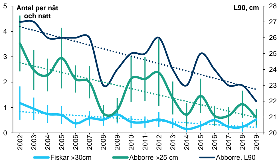
Figur 5. Fångst per nät och natt av stora individer och stora abborrar. Vertikala linjer anger 95 % konfidensintervall. Streckade linjer anger statistiskt säkerställda trender över tid.
