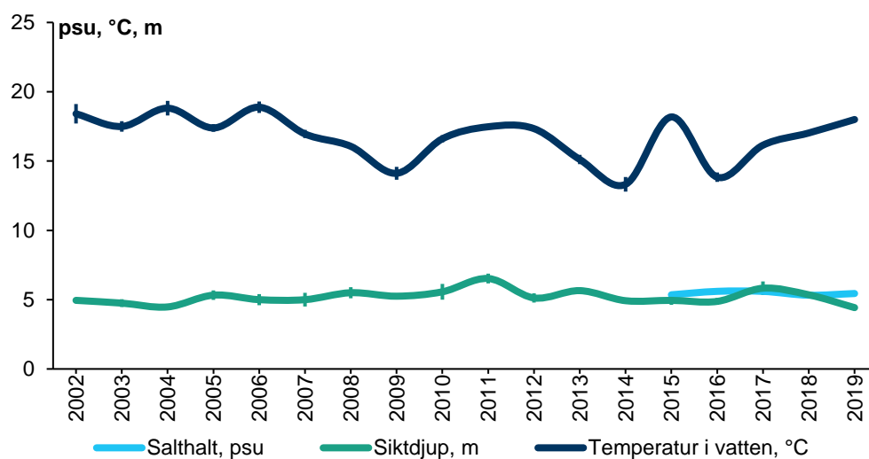
Figur 2. Temperatur, siktdjup och salthalt (medelvärden) vid vittjning av provfiskefångsten. Temperatur och salthalt mäts i bottenvattnet vid varje station. Vertikala linjer anger 95 % konfidensintervall.
