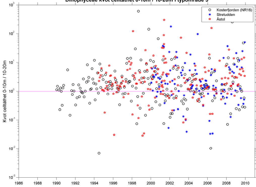
Dinophyceae kvot cellt tthet 0-10m / 10-20m i typomr de 3
