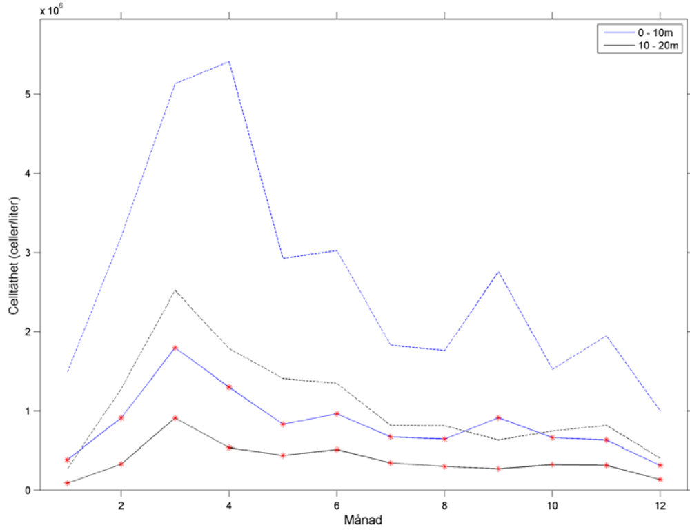
Medelcelltäthet, 0-10m och 10-20m med +STD (-STD hamnar under 0)
