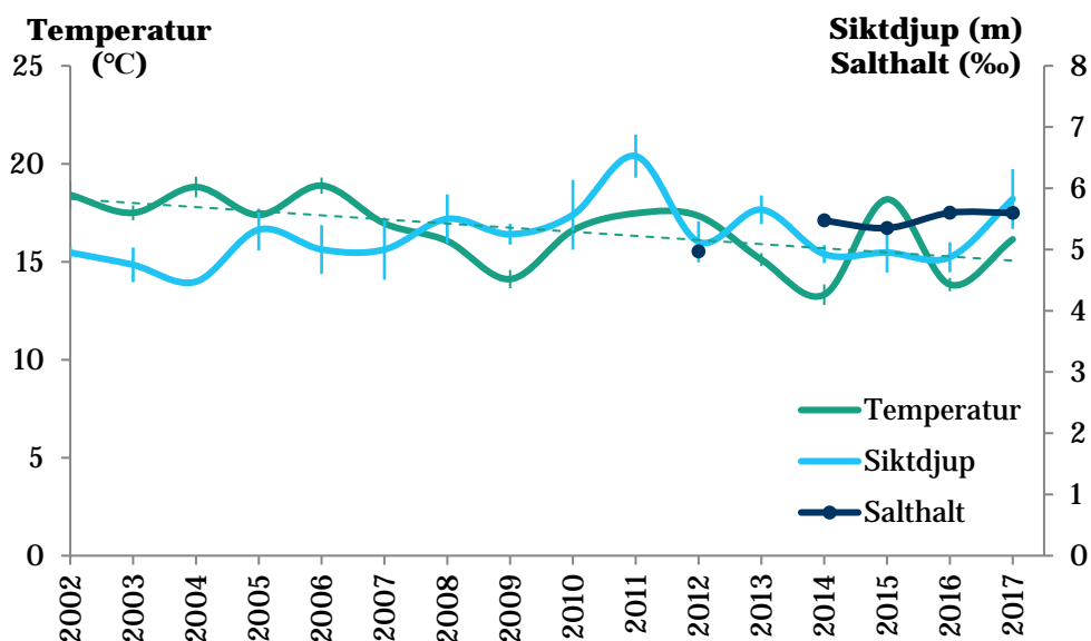
Figur 1. Temperatur, siktdjup och salthalt (medelvärden) vid vittjning av provfiskeät. Temperatur och salthalt mäts i bottenvattnet vid varje station. Vertikala linjer anger 95 % konfidensintervall. Streckad linje anger statistiskt säkerställd trend över tid.
