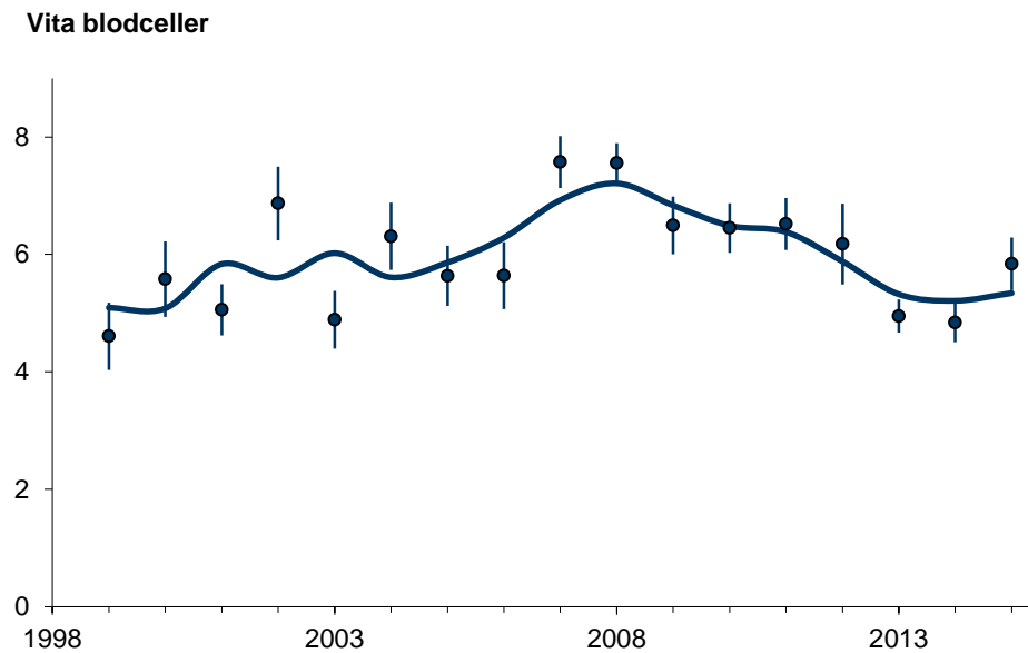
Figur 16. Totala andelen vita blodceller (% av totalt antal blodceller) i blodet hos abborrhonor. Vertikala linjer anger 95 % konfidensintervall. Den grövre linjen visar tre års glidande medelvärde.
