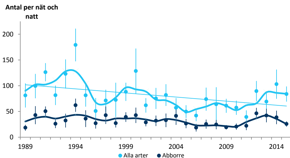
Figur 2. Fångst (antal per station) av alla arter och abborrar under provfiske i augusti. Vertikala linjer anger 95 % konfidensintervall. De grövre linjerna visar tre års glidande medelvärde. Tunna linje visar signifikant trend.
